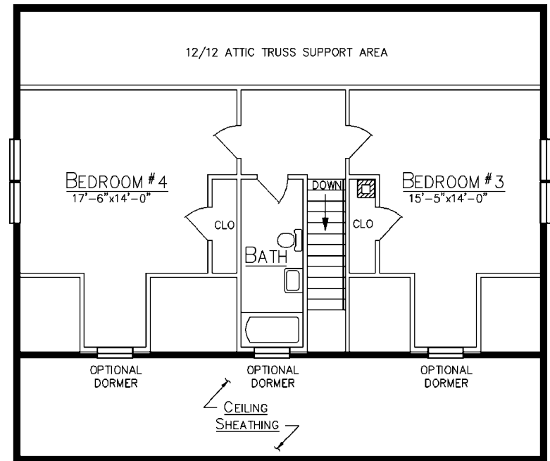
LOFT PLAN
