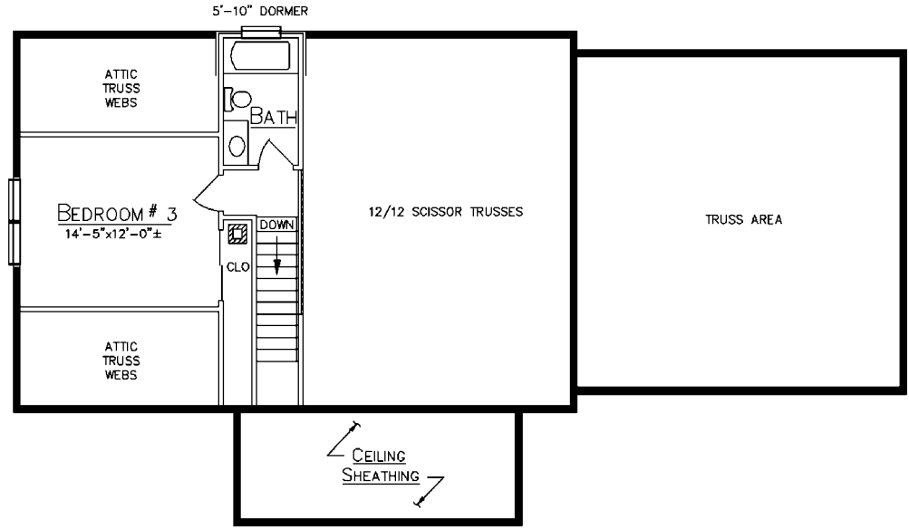
LOFT PLAN
