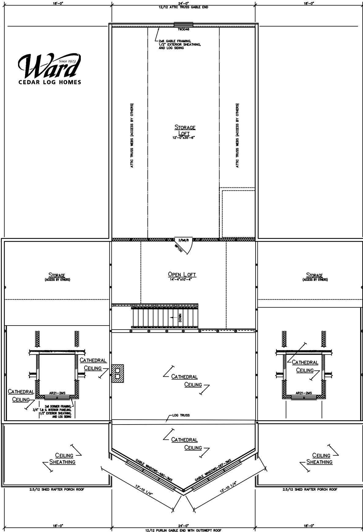
LOFT PLAN
